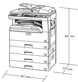
Obrázek stroje s doplňky.
